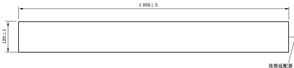
图7 用于耦合夹校准的感应板
